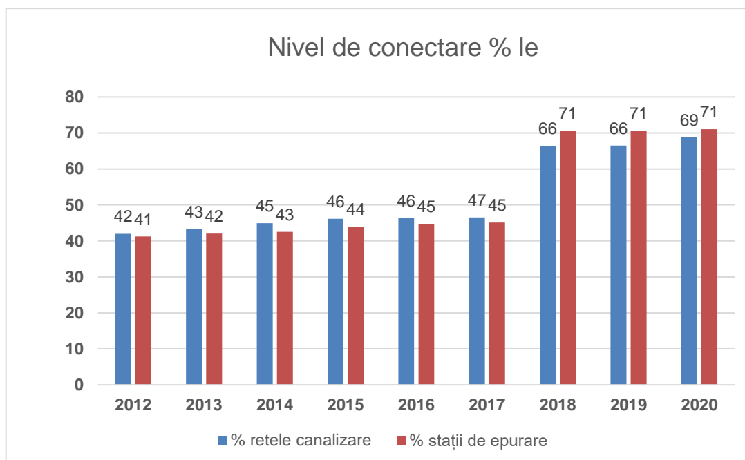
Figura 9.2 Progresul anual înregistrat pentru colectarea și epurarea apelor uzate urbane, în aglomerări mai mari de 2.000 l.e.
