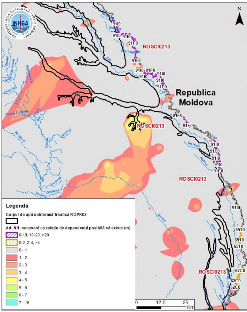
Figura 4.8 Variația amplitudinii adâncimii nivelului hidrostatic în perioada 2000-2017, în zona sitului de importanță comunitară ROSCI0213
