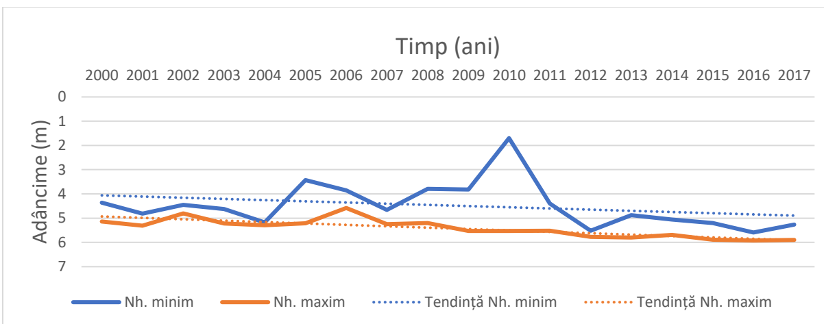
Figura 4.5 Variația adâncimii minime și maxime anuală a nivelului hidrostatic (m) măsurată față de cota terenului, în perioada 2000-2017, în forajul F1 Cârniceni, situat în cadrul sitului ROSCI0213, aparținând corpului de apă subterană freatică ROPR02
