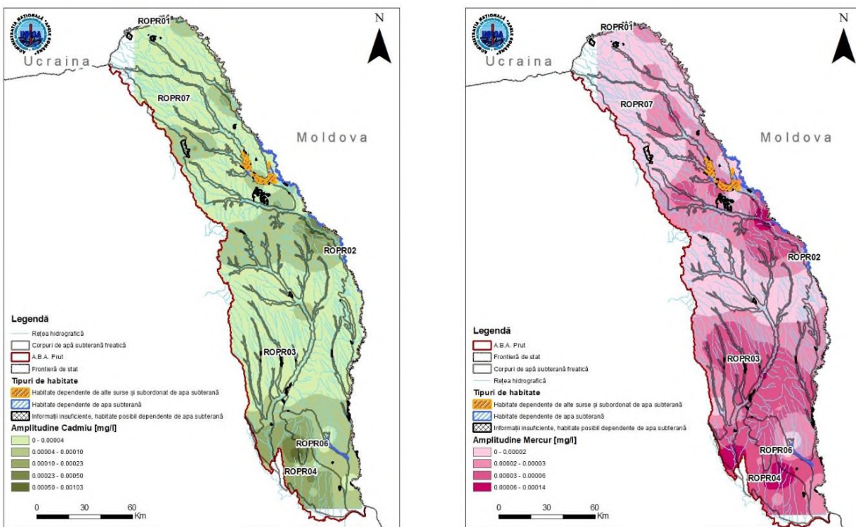
Figura 4.20 Variația diferenței dintre valoarea maximă și minimă a parametrilor chimici cadmiu (A) și mercur (B) în arealul habitatelor dependente de subterană
