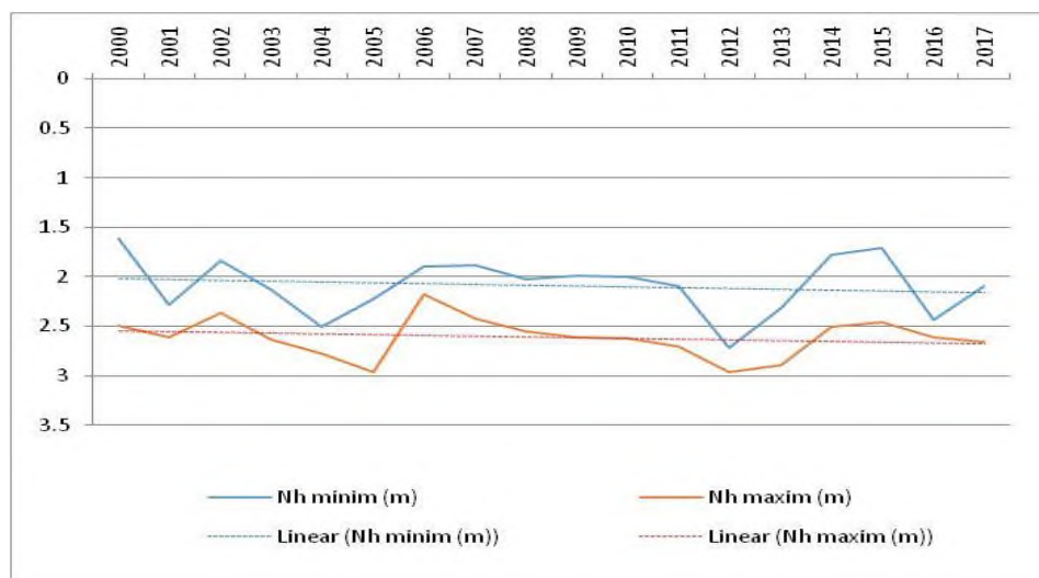
Figura 4.9 Variația adâncimii minime și maxime anuală a nivelului hidrostatic (m) măsurată față de cota terenului, în perioada 2000-2017, în forajul F3 Cârniceni, situat pe sitului ROSCI0222, aparținând corpului de apă subterană freatic ROPR02
